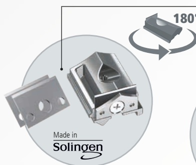
Регулируемый блок лезвия можно повернуть на 180 градусов при необходимости.
